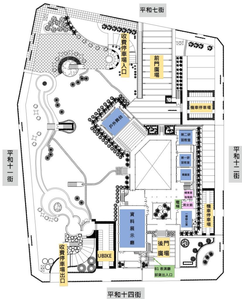
一樓平面圖
